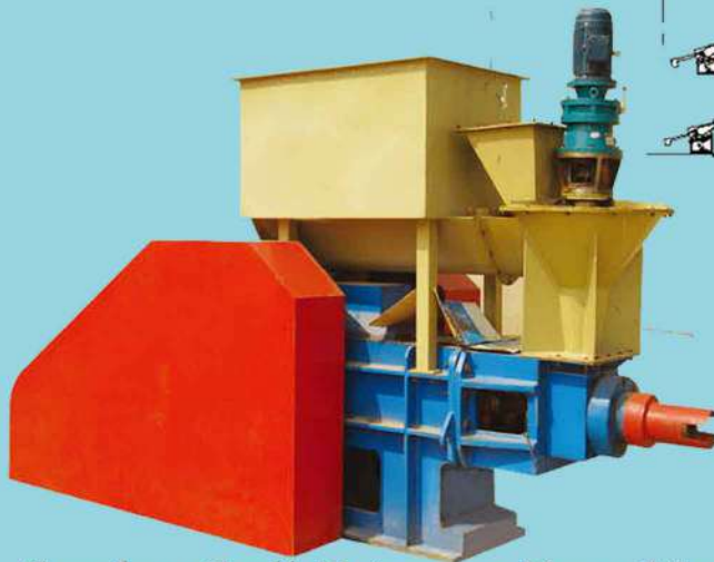
Sawdust Stalk Briquette Press Machine
